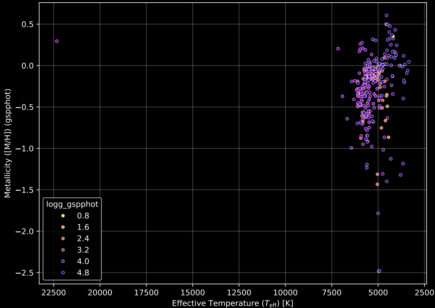
APOGEE DR17 Field: [M68] Stellar Population Parameters (n= 271)
